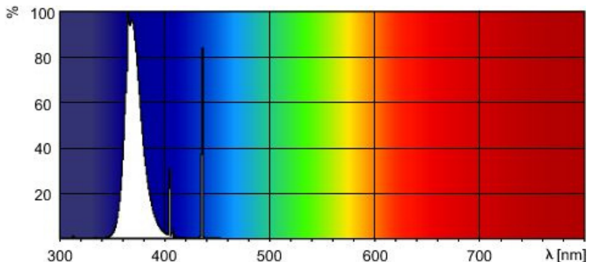
Phân bố công suất phổ – đèn TL 80W/10-R SLV/25
