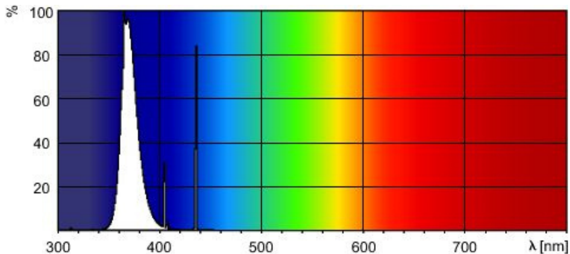
Phân bố công suất phổ – đèn TL 60W/10-R SLV/25
